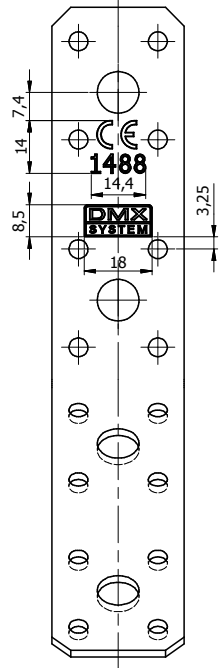
Widok A
